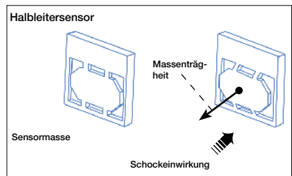
Airbagsteuergerät mit integrierten Sensoren
