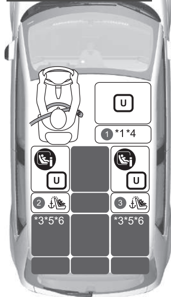
Beifahrer-Airbag ausgeschaltet für Linkslenker-Ausführung
