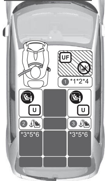
Beifahrer-Airbag eingeschaltet für Linkslenker-Ausführung
