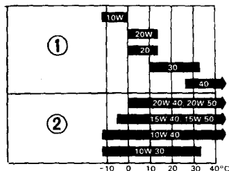
(1) Einbereichsöl
