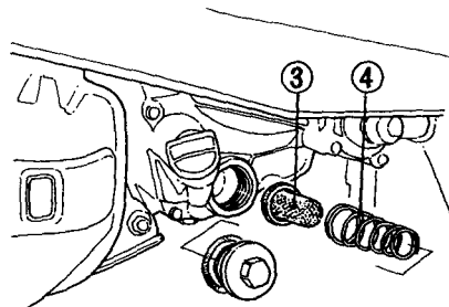
(3) Ölsieb
