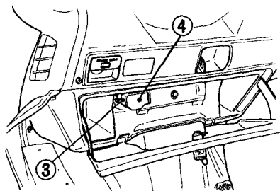
(3) Sicherungskasten (4) Sicherungskastendeckel
