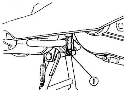
(1) Tappo scarico
