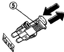
(5) Estrattore fusibili
