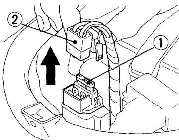
(1) Hauptsicherung
