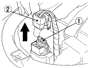
(1) Fusibile principale
