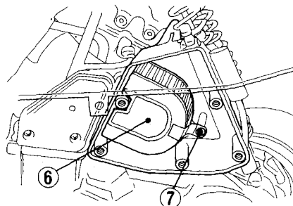
(6) Luftfilterelement (7) Schraube
