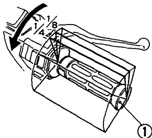
(1) Gasdrehgriff
