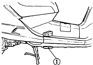
(1) Rahmennummer
